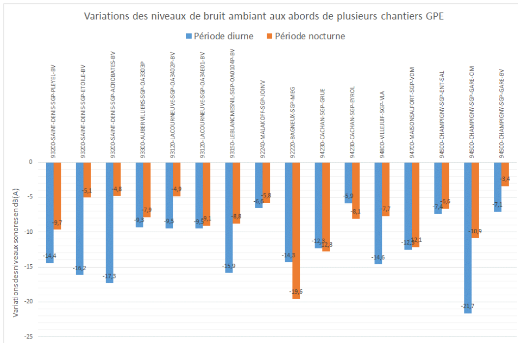
Variations des niveaux de bruit ambiant diurne et nocturne entre après et avant l'arrêt des chantiers sur plusieurs stations de mesure de Bruitparif situées aux abords de chantiers de construction du Grand Paris Express
