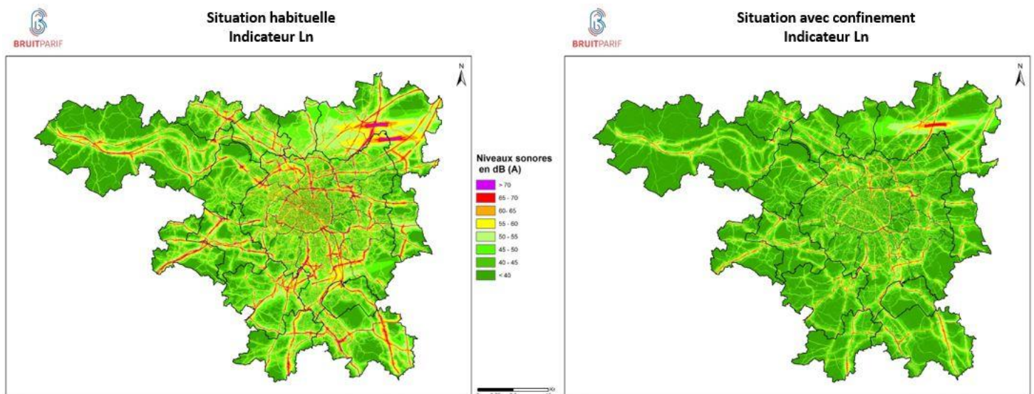
Cumul des bruits liés aux trafics routier, aérien et ferroviaire au sein de la zone dense francilienne. Indicateur Ln
